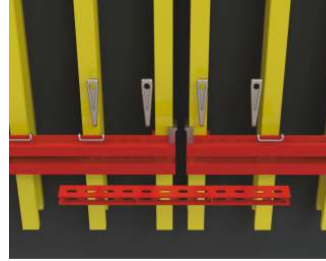
Portiwood kuşak birleştirme elemanı ve kaması ile daha geniş paneller elde edilebilir. Wider panels can be obtained with the Portiwood waler and wedge.
